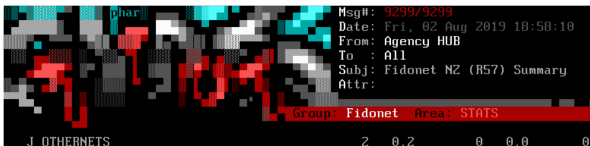
Fig. 19. ANSI-арт
