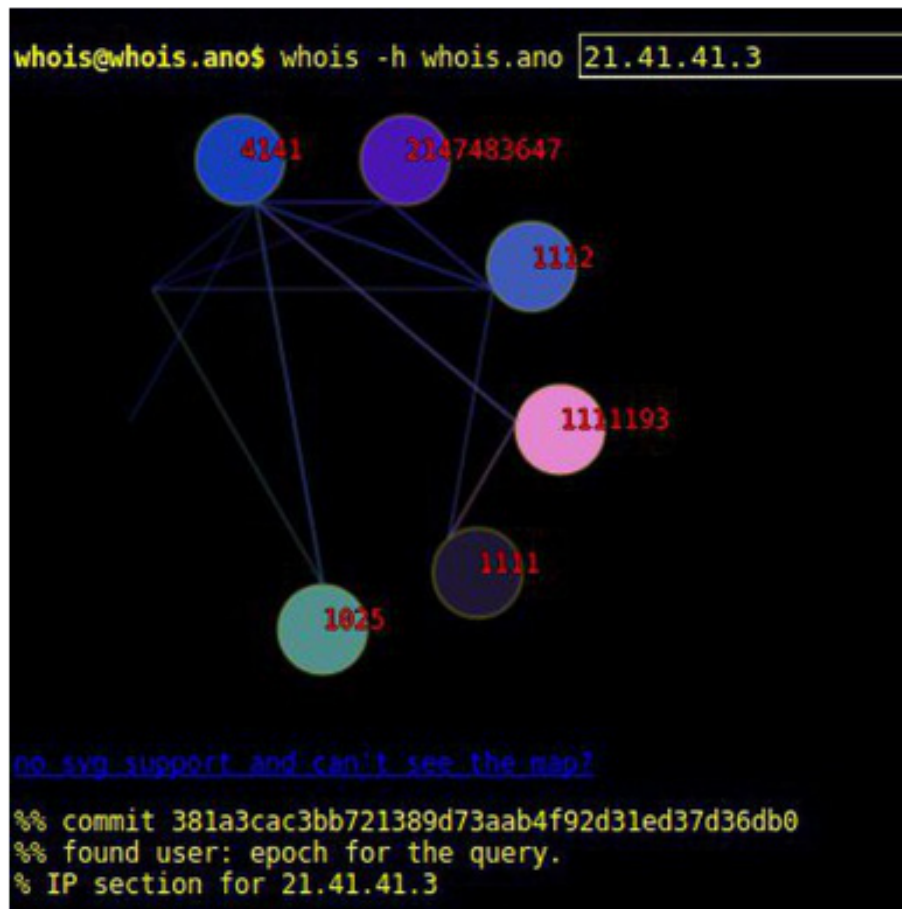
Fig. 9. структура Анонета
